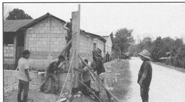
Foto 4: FUNDICION DE COLUMNA EN LA ESQUINA DEL CERCO PERIMETRAL PARA TENER UNA MEJOR RESISTENCIA DE LAS MALLAS.
